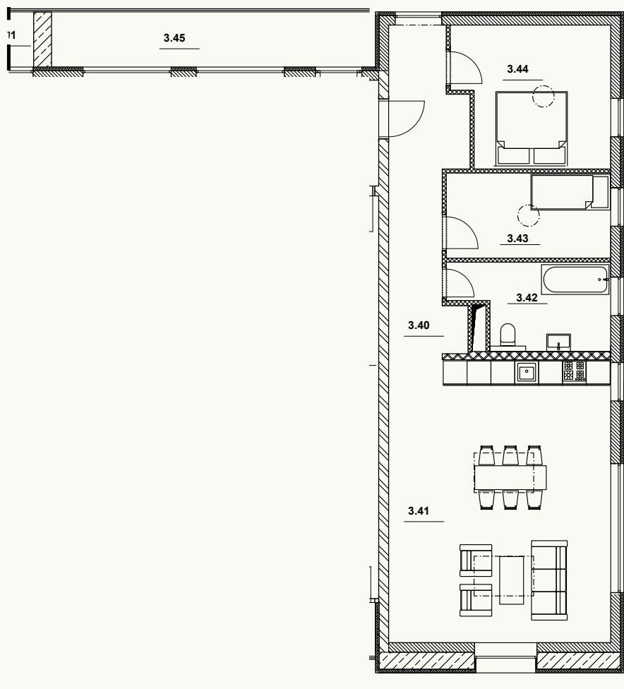
UMÍSTĚNÍ BYTU V PŮDORYSU 3. NP
