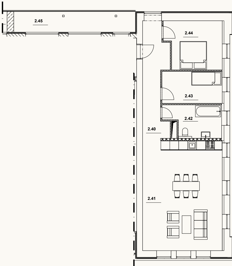
UMÍSTĚNÍ BYTU V PŮDORYSU 2. NP
